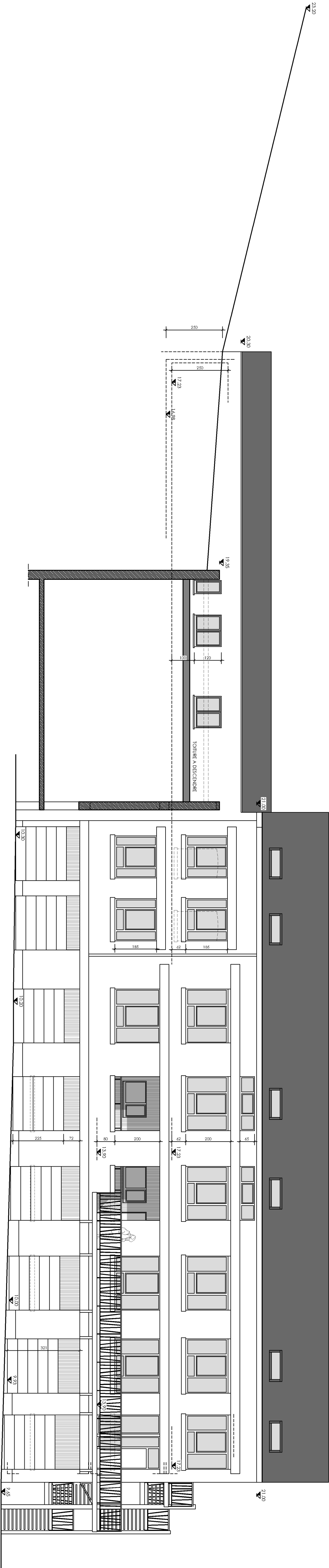
COUPE CC
