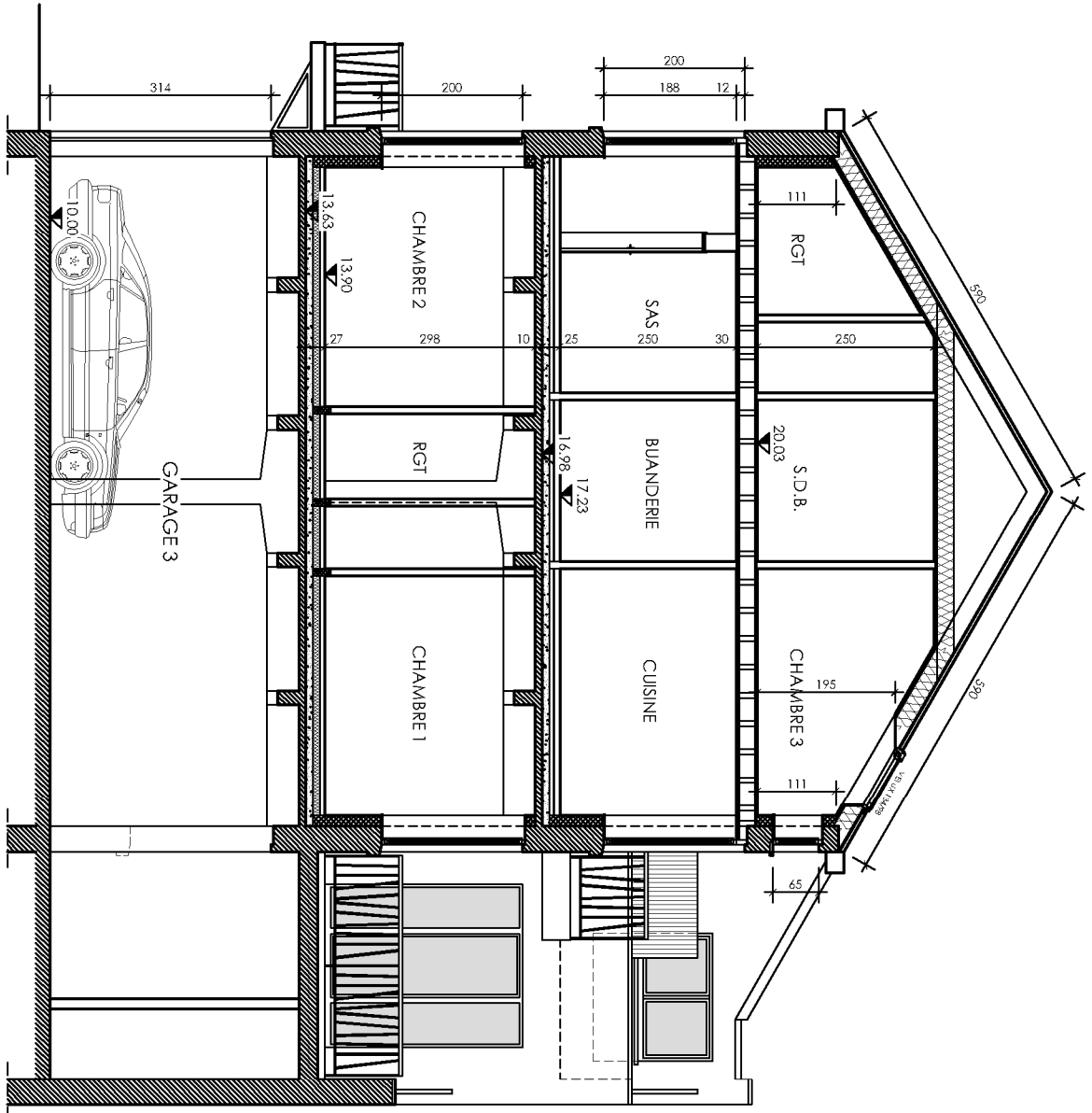
COUPE AA
