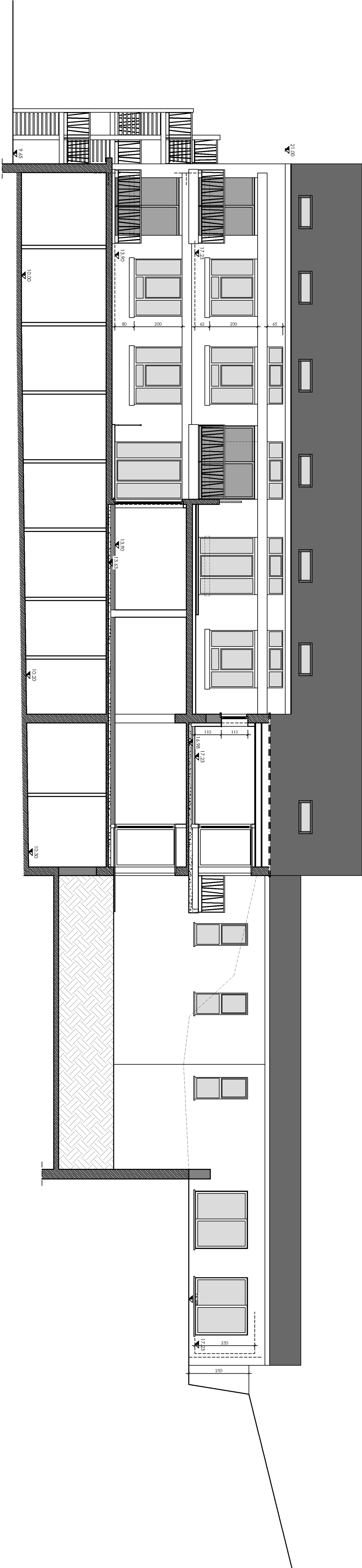
COUPE BB
